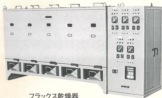
フラックス乾燥器 GF-10-5PR
